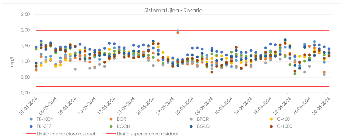
Gráfico 5-9 Resultados parámetros tipo V – cloro libre residual, Sistema Ujina y Rosario.
