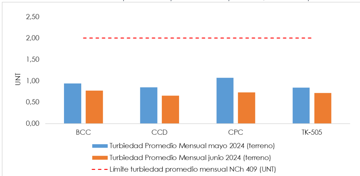
Gráfico 5-3 Resultados parámetros tipo I - turbiedad promedio, Sistema Coposa
