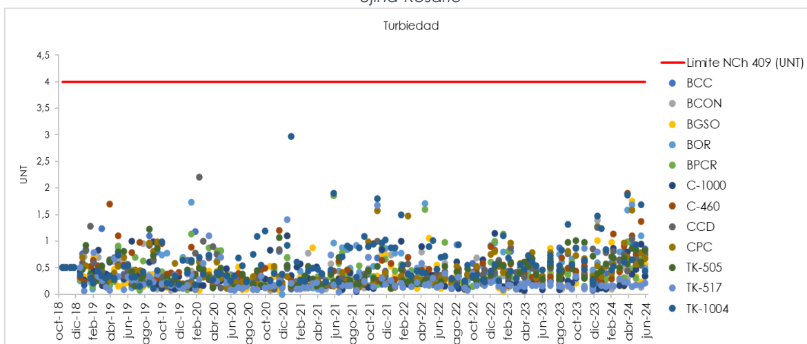
Gráfico 6-2 Resultados históricos de turbiedad (noviembre 2018 – junio 2024) Sistemas Coposa y Ujina-Rosario
