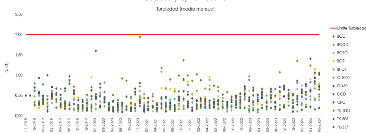
Gráfico 6-3 Resultados históricos de turbiedad media mensual (noviembre 2018 – junio 2024) Sistemas Coposa y Ujina-Rosario.
