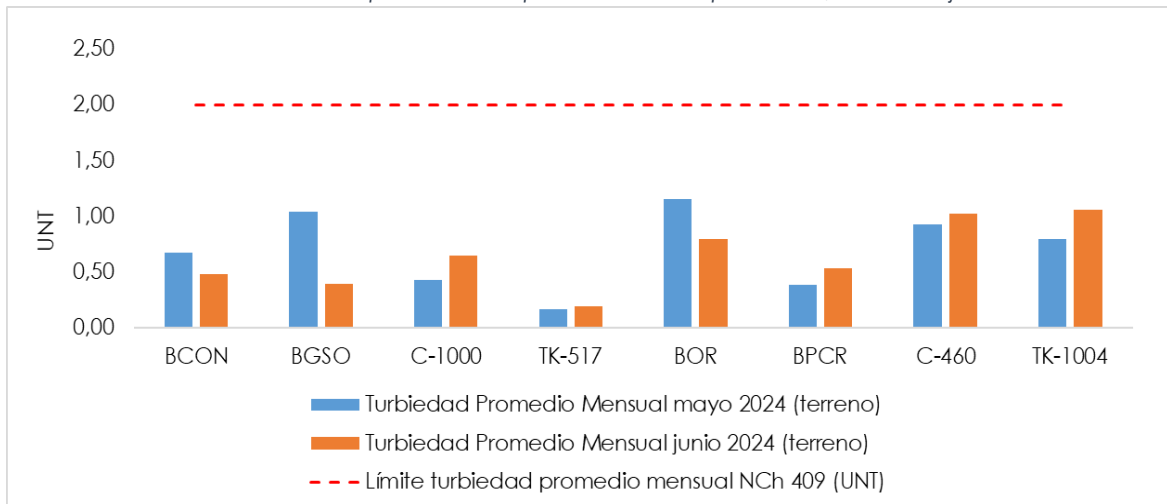
Gráfico 5-8 Resultados parámetros tipo I - turbiedad promedio, Sistema Ujina-Rosario.
