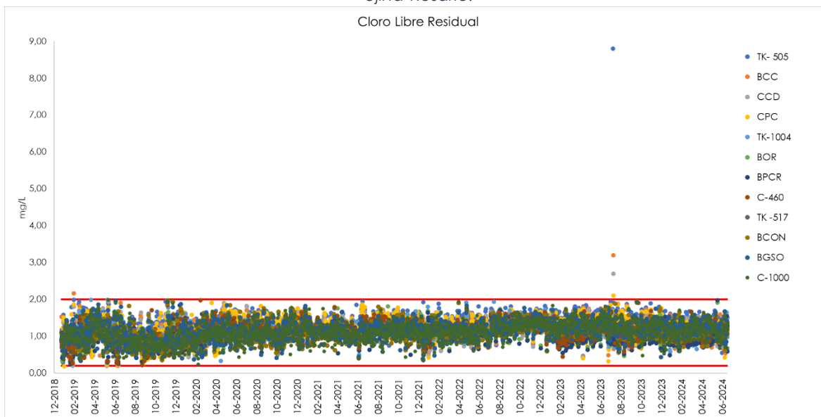
Gráfico 6-4 Resultados históricos de cloro libre residual (enero 2019 – junio 2024) Sistemas Coposa y Ujina-Rosario.
