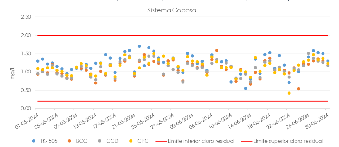
Gráfico 5-4 Resultados parámetros tipo V – cloro libre residual, Sistema Coposa.
