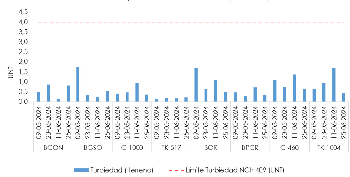
Gráfico 5-7 Resultados parámetros tipo I – turbiedad, Sistema Ujina-Rosario.
