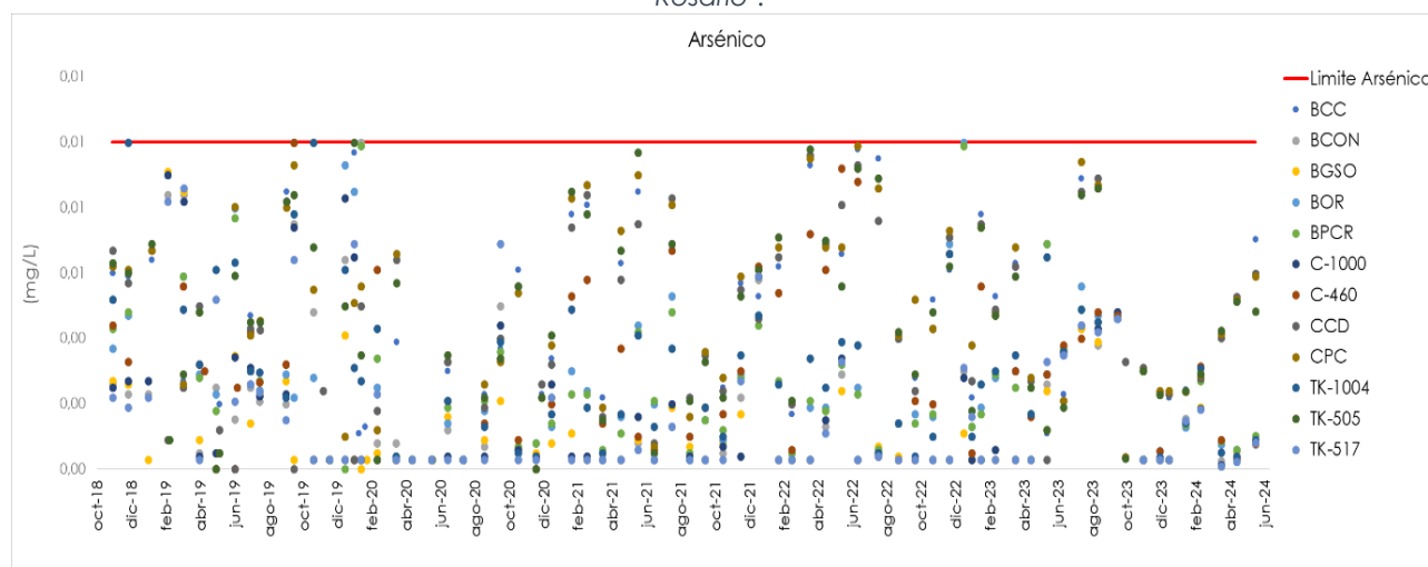
Gráfico 6-5 Resultados históricos Arsénico (noviembre 2018 – junio 2024) Sistemas Coposa y Ujina-Rosario 8 .
