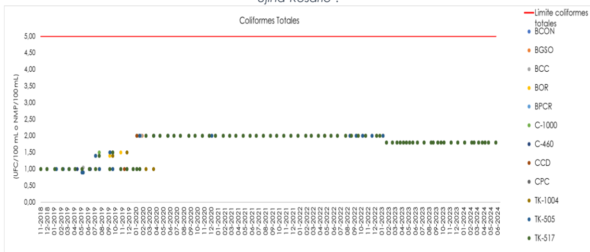
Gráfico 6-1 Resultados históricos coliformes totales (noviembre 2018 – junio 2024) Sistemas Coposa y Ujina-Rosario 7 .
