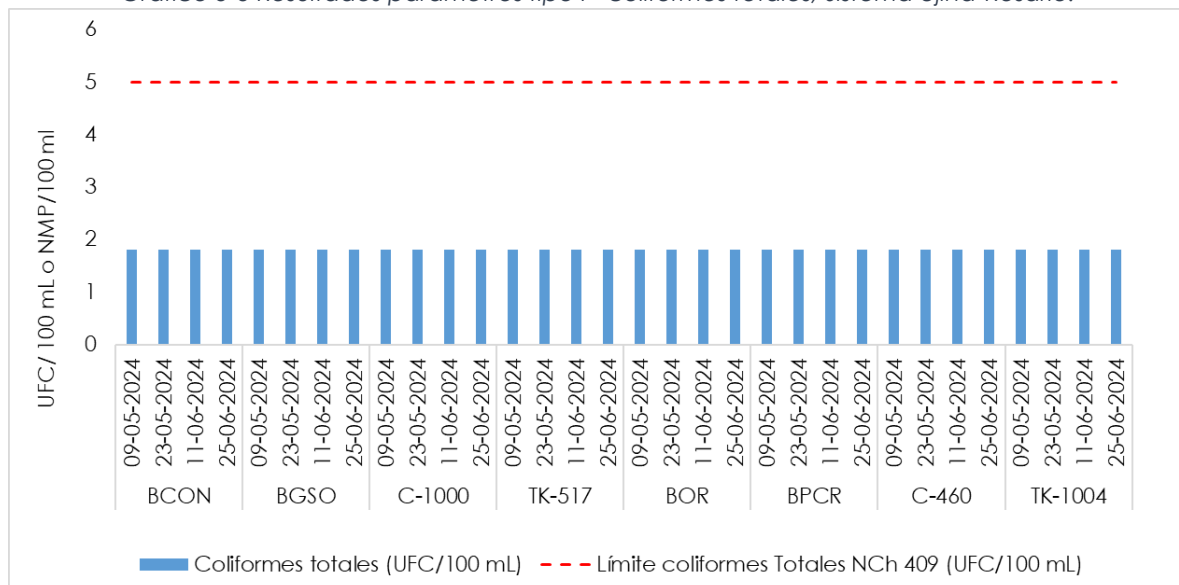
Gráfico 5-6 Resultados parámetros tipo I - coliformes totales, Sistema Ujina-Rosario.
