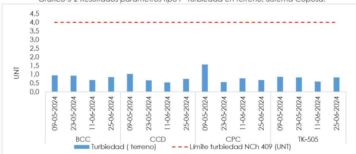
Gráfico 5-2 Resultados parámetros tipo I - turbiedad en terreno, Sistema Coposa.
