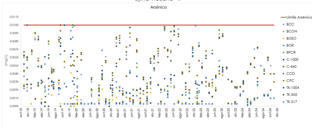
Gráfico 6-5 Resultados históricos arsénico (noviembre 2018 – diciembre 2024) Sistemas Coposa y Ujina-Rosario 13 .
