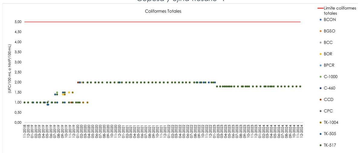
Gráfico 6-1 Resultados históricos coliformes totales (noviembre 2018 – diciembre 2024) Sistemas Coposa y Ujina-Rosario 12 .
