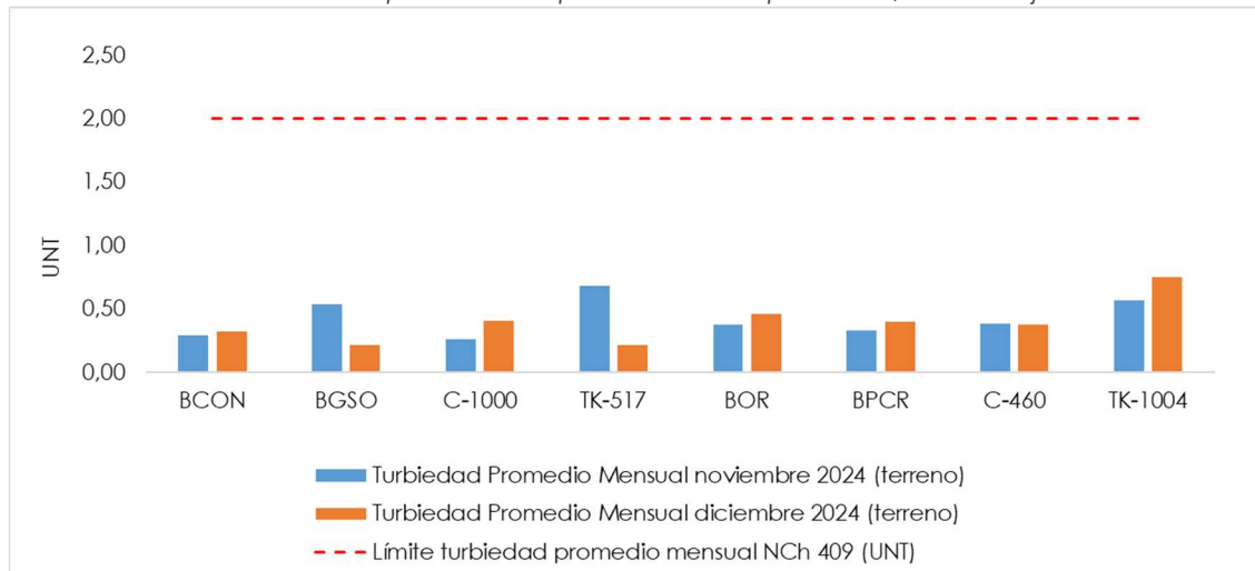
Gráfico 5-8 Resultados parámetros tipo I - turbiedad promedio, Sistema Ujina-Rosario.
