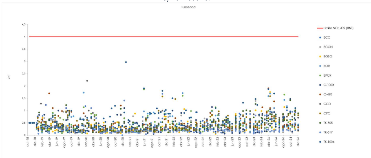
Gráfico 6-2 Resultados históricos de turbiedad (noviembre 2018 – diciembre 2024) Sistemas Coposa y Ujina-Rosario.
