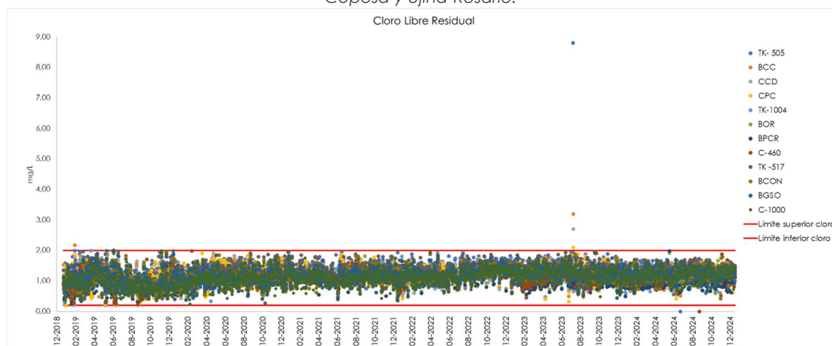
Gráfico 6-4 Resultados históricos de cloro libre residual (enero 2019 – diciembre 2024) Sistemas Coposa y Ujina-Rosario.
